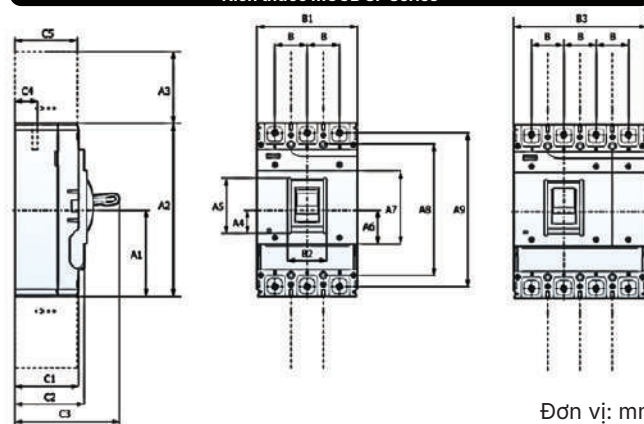
Kích thước MCCB SF Series
