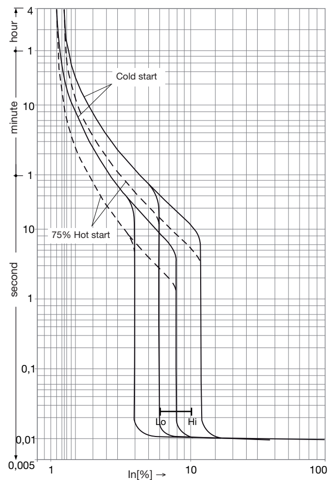
MCCB h800 TM (630A)
