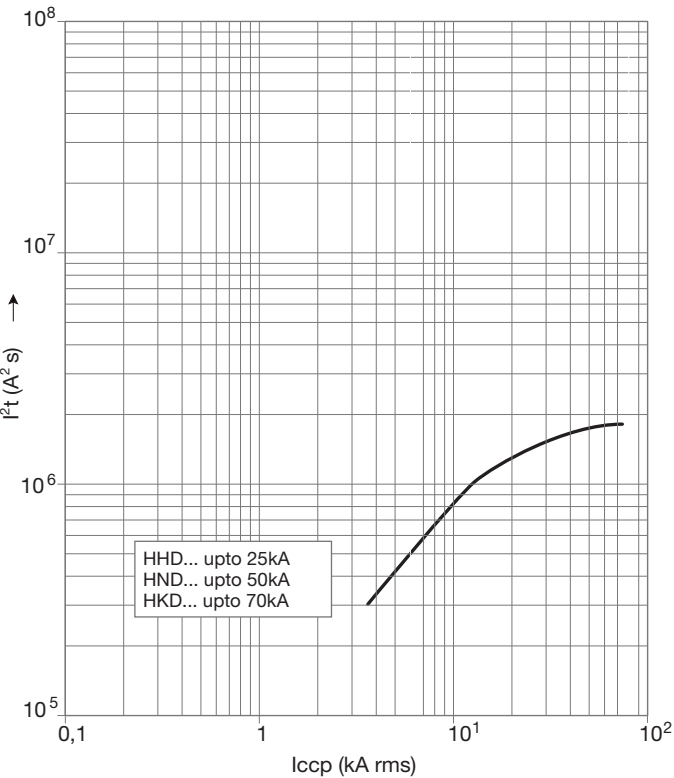
MCCB h400 TM (250A)
