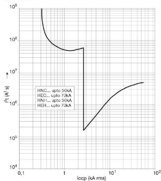
MCCB h250
