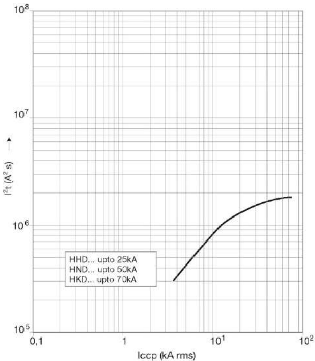
MCCB h400 TM (250A)
